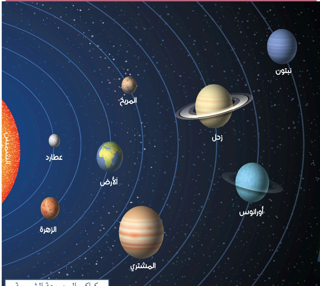
كواكب المجموعة الشمسية
